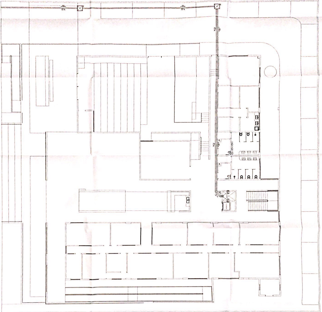
PLANTA SALA 1º PAVIMENTO Esc.: 1:75
